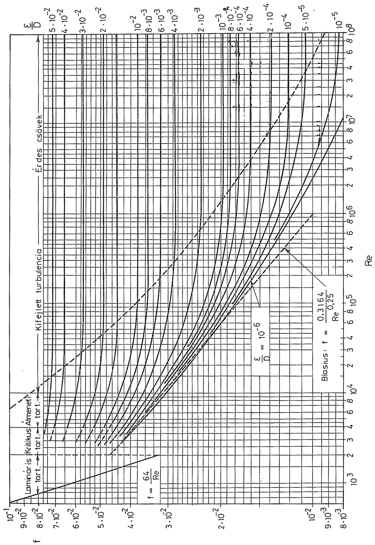
9.3. ábra Súrlódási tényező érdes csövekben
